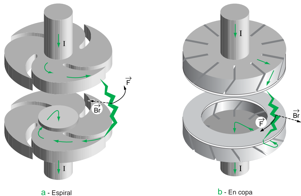
Fig. 10: Estructuras de contactos utilizados para crear el campo radial (espiral y copa «contrate»).
