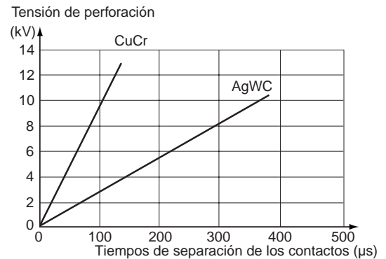
Fig. 23: Evolución de la rigidez dieléctrica entre contactos a partir del instante de su separación, según el tipo de material.
